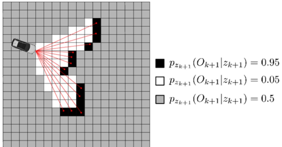
Şekil 4.5 2B Occupancy Grid Doluluk Haritası
